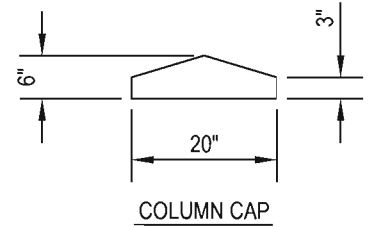
COLUMN CAP
